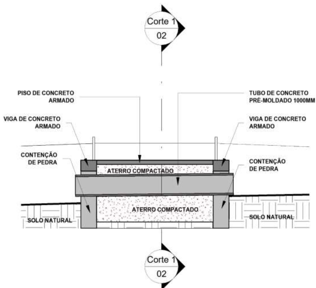
CORTE 02
